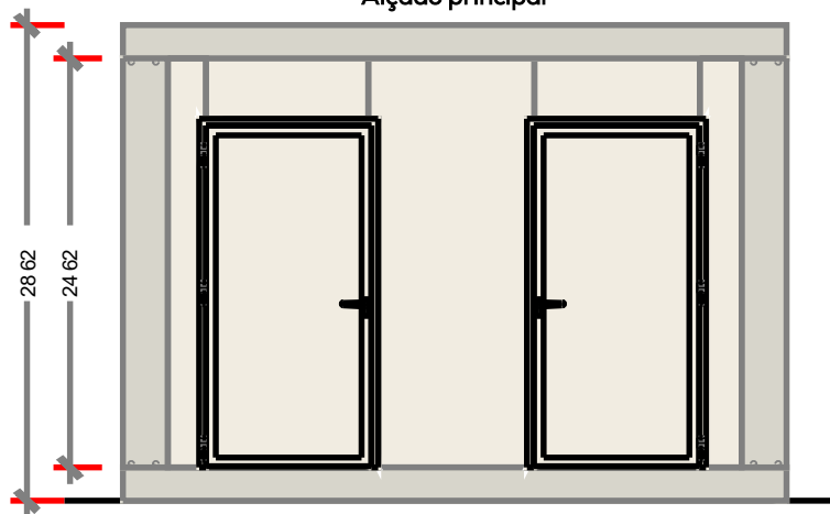
Alçado principal
