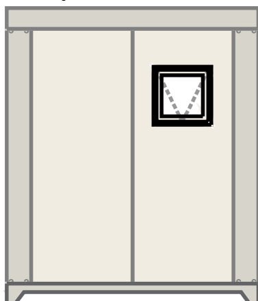
Alçado lateral esquerdo
